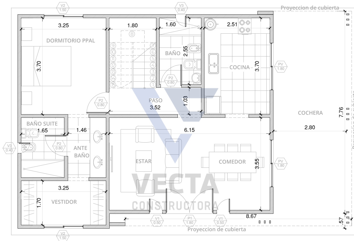
PLANTA BAJA
